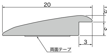
断面図 (単位: mm)
